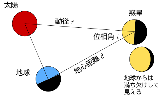
図 1: 惑星の等級
